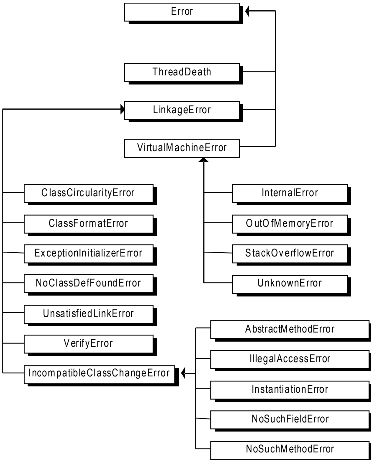
Рисунок 5. Потомки класса Error
