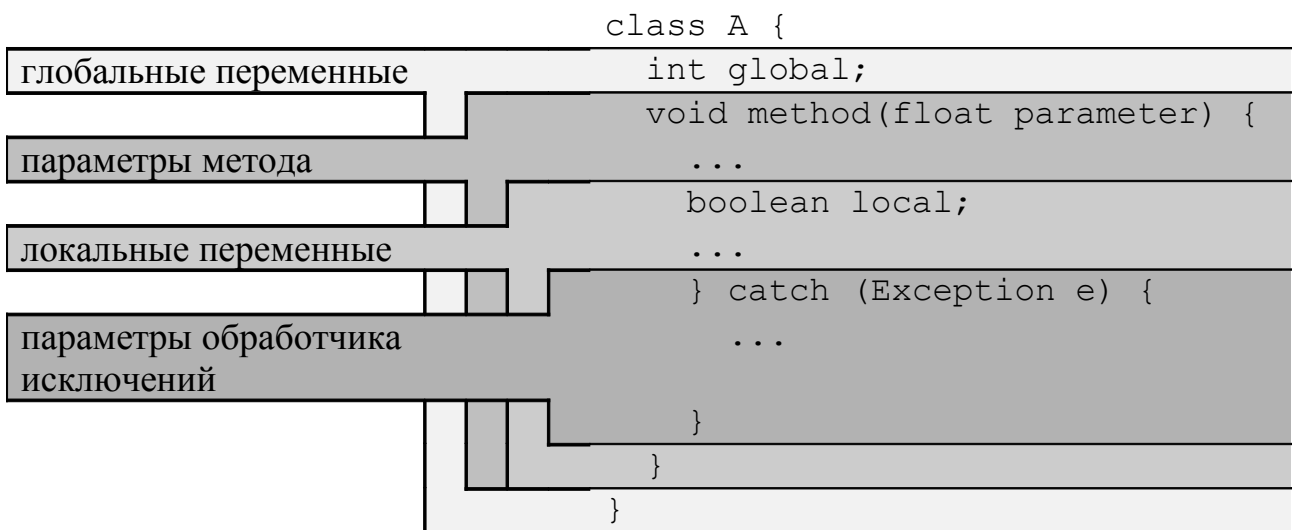
Рисунок 1. Области видимости переменных
