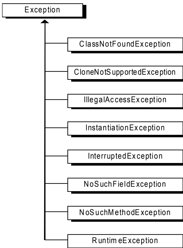
Рисунок 3. Исключения пакета java.lang
